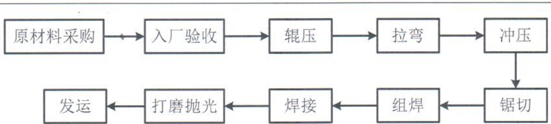
图1 车门框加工生产工艺流程图
